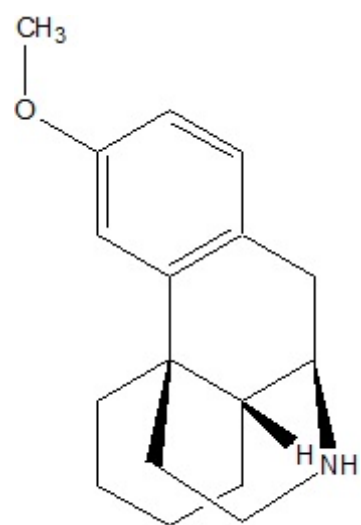
3-Methoxymorphinan
